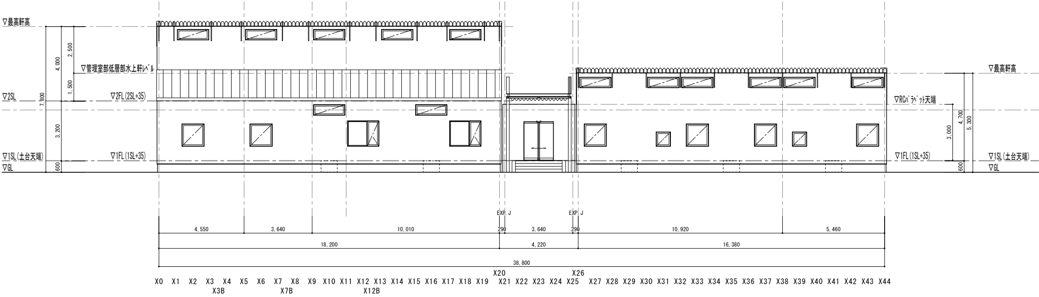
南立面図 S=1:200
