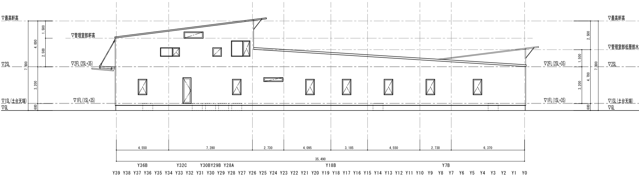
西立面図 S=1:200
