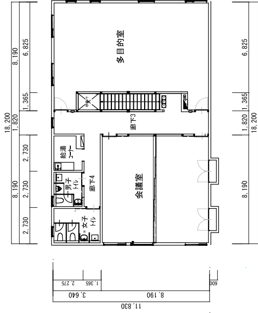
2階平面図
