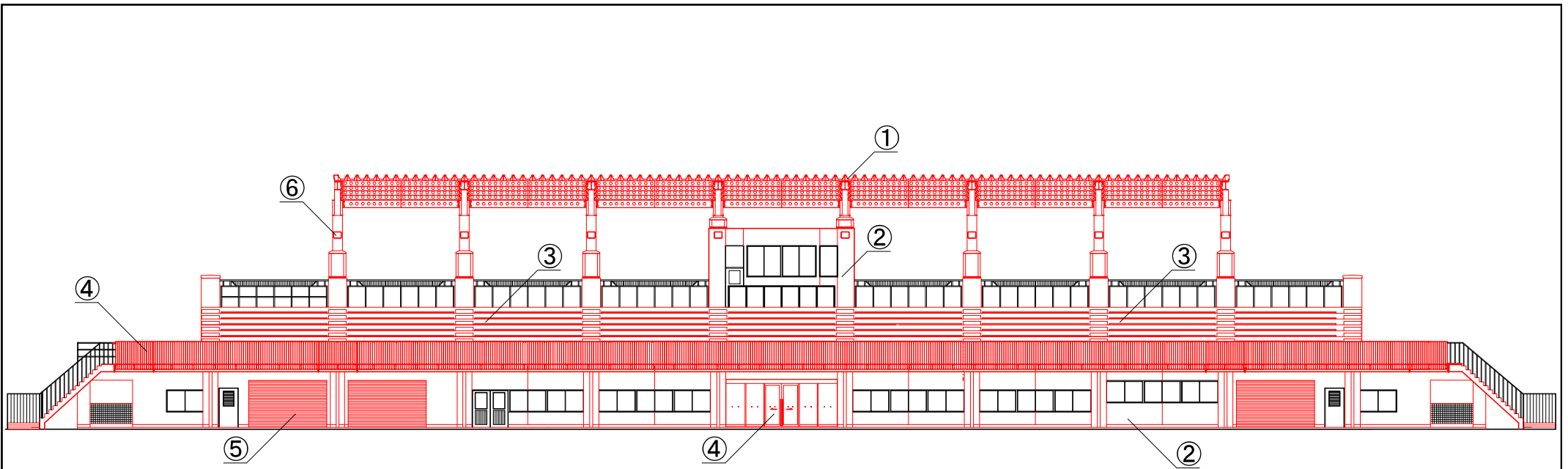
南側立面図
