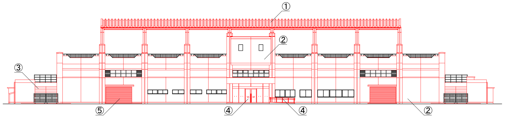
北側立面図
