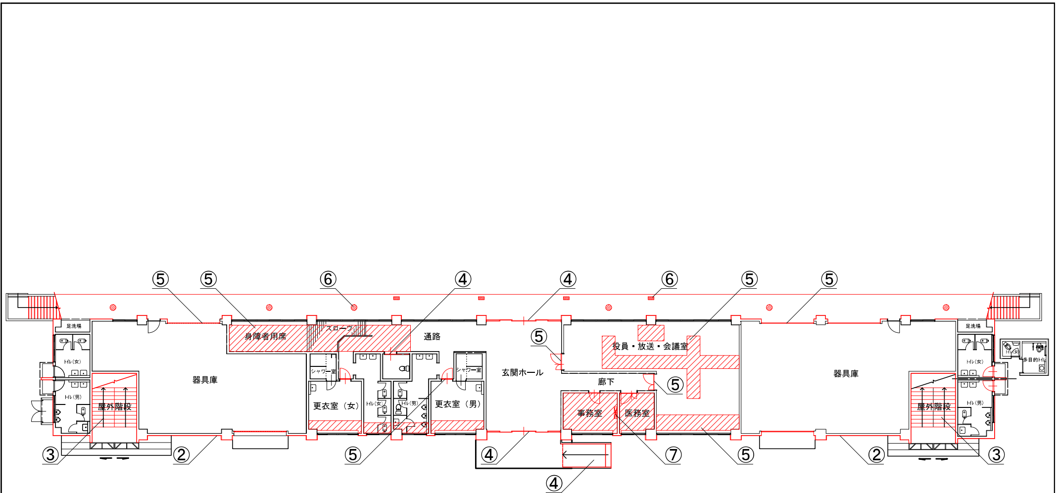
平面図（1階）
