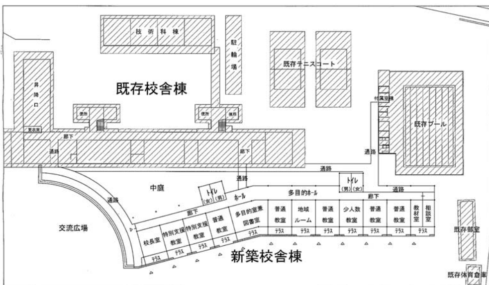
(仮称)長狭地区小中一貫校の平面図
