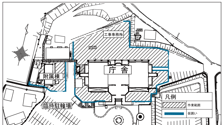
庁舎の作業範囲と仮囲い
