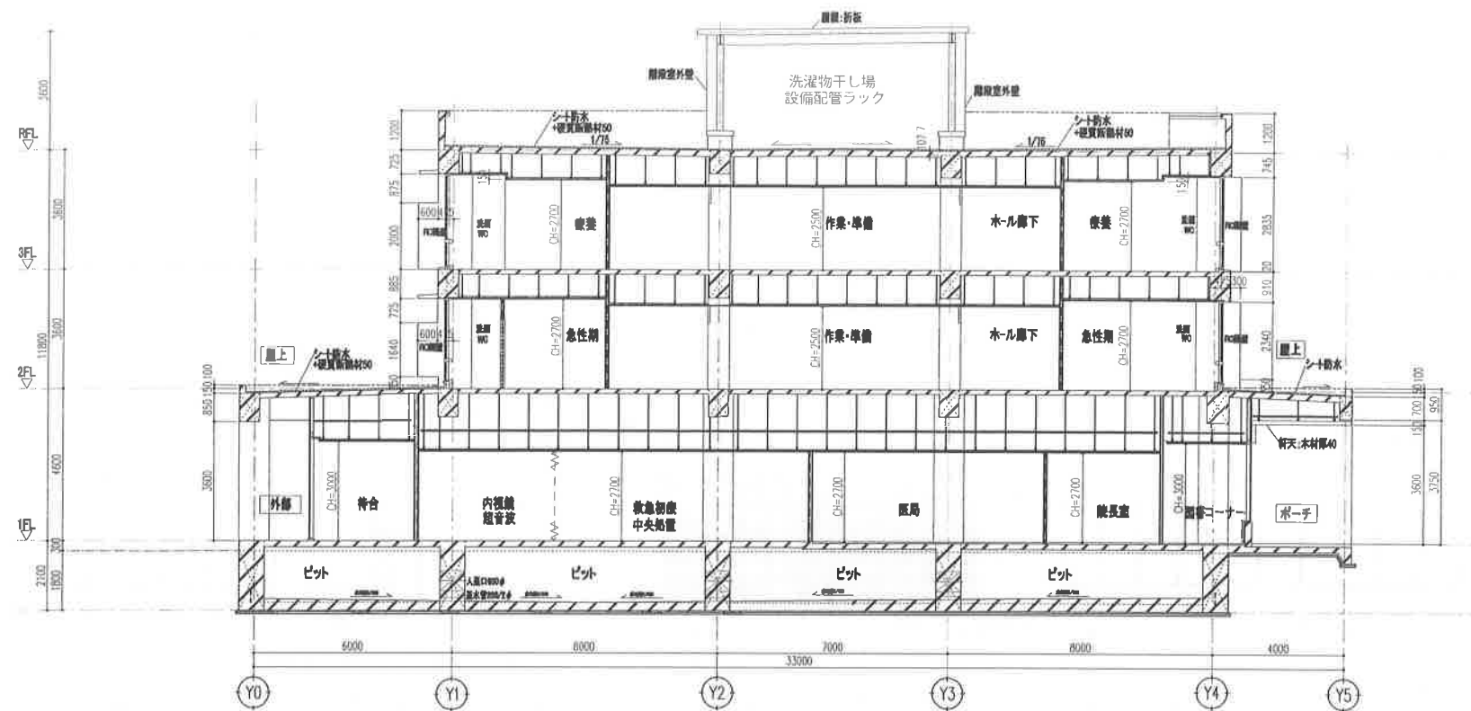
Y方向断面図 (X6位置)
