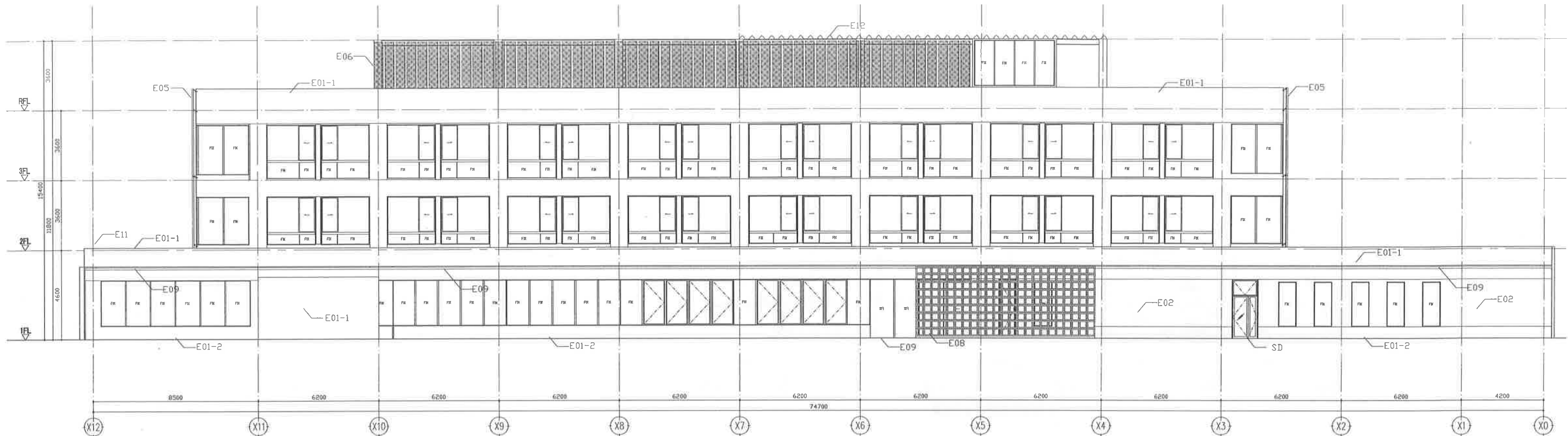
北立面図
