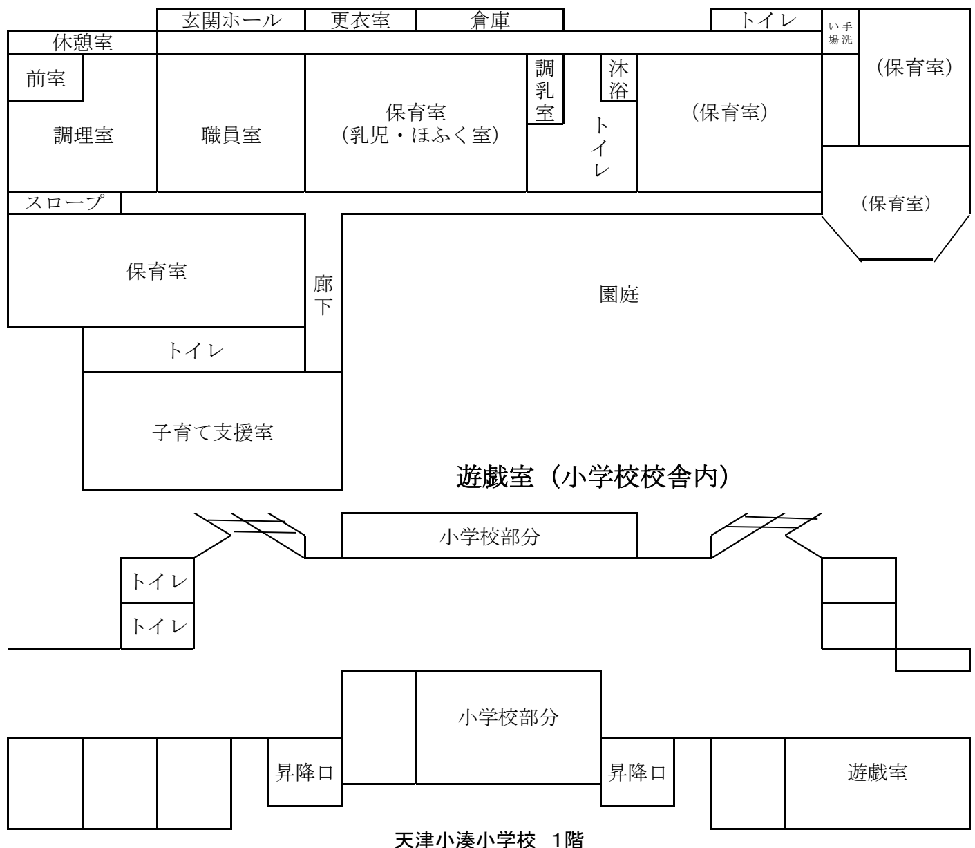
天津小湊認定こども園平面図
