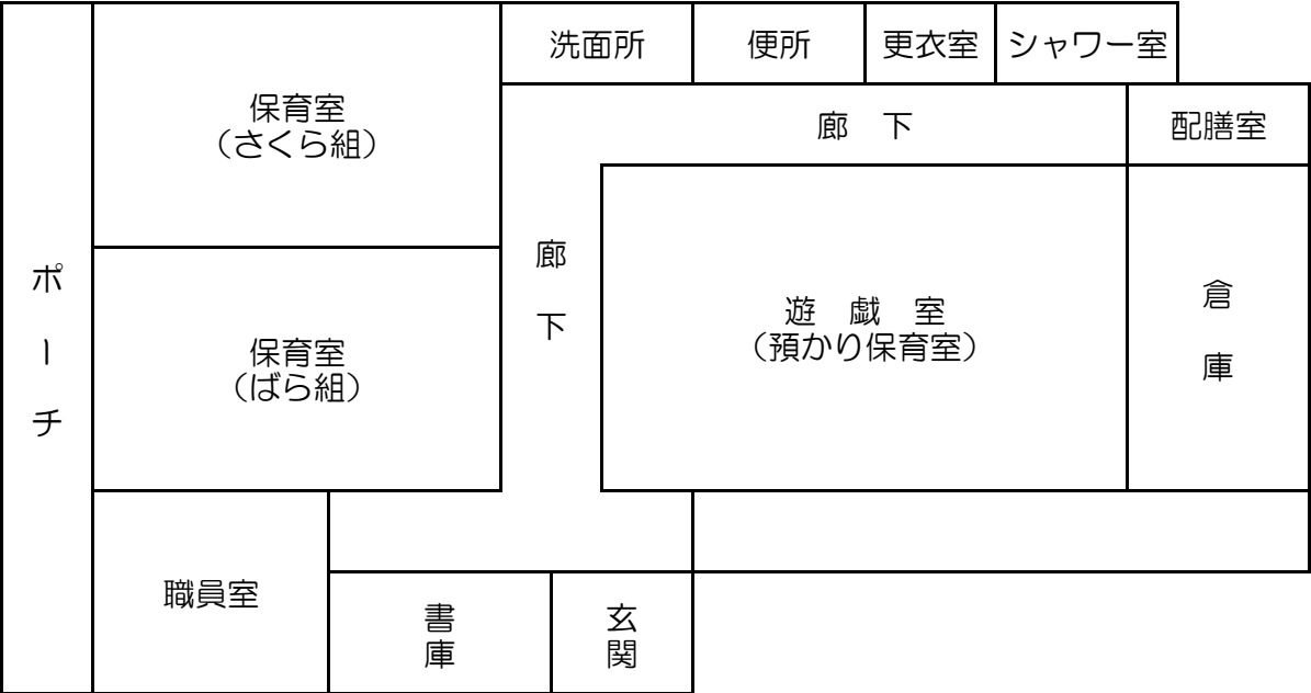
田原認定こども園平面図(さくら棟)
